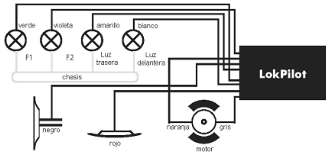
Fig. 2 – Cableado del LokPilot con el polo común conectado al chasis
